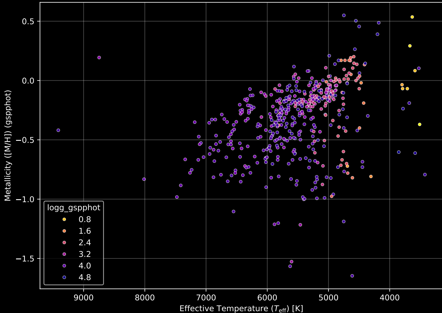
GALAH DR4 Field: [6785] Stellar Population Parameters (n= 462)
