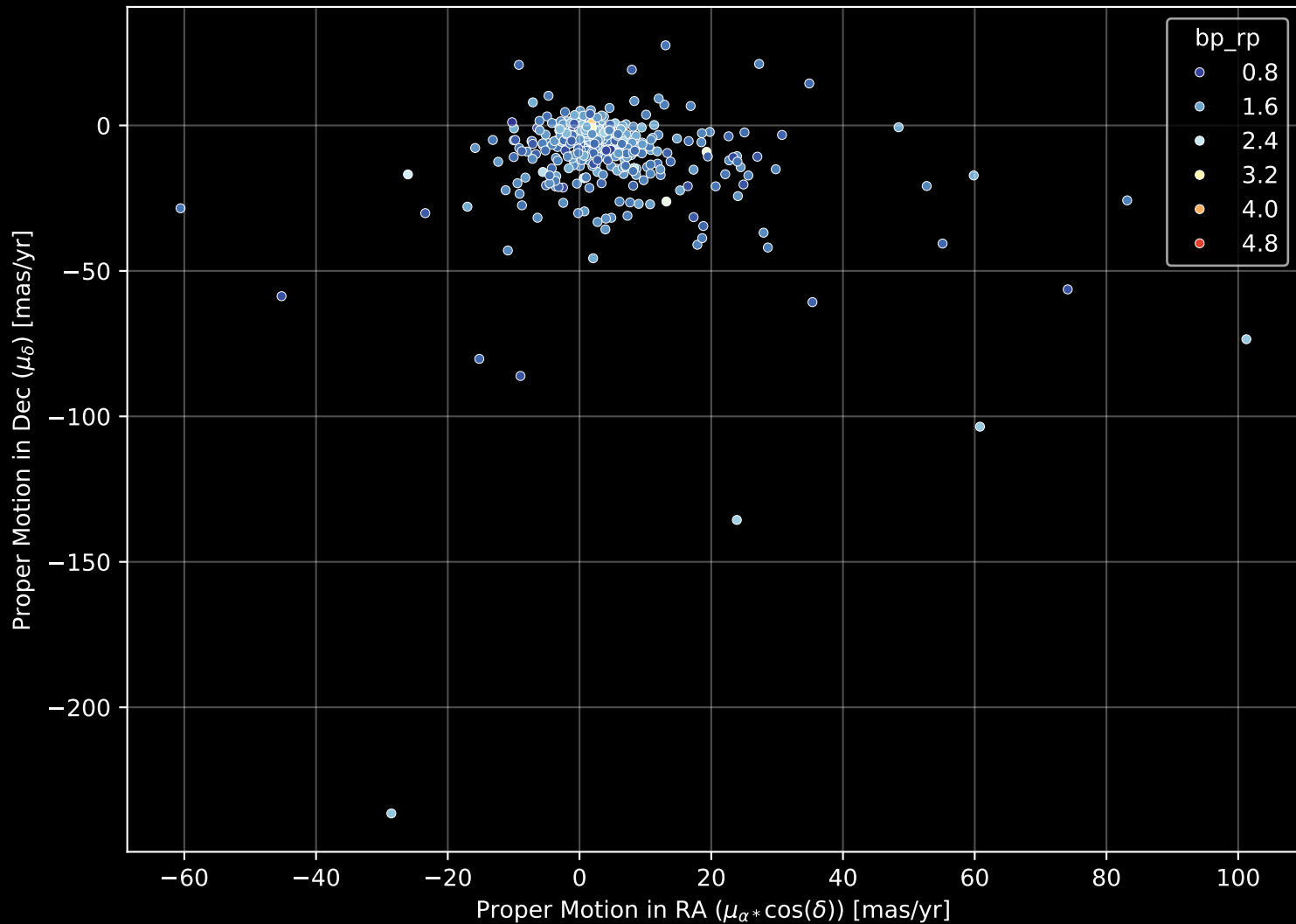
GALAH DR4 Field: [6785] Proper Motion Diagram (n= 462)
