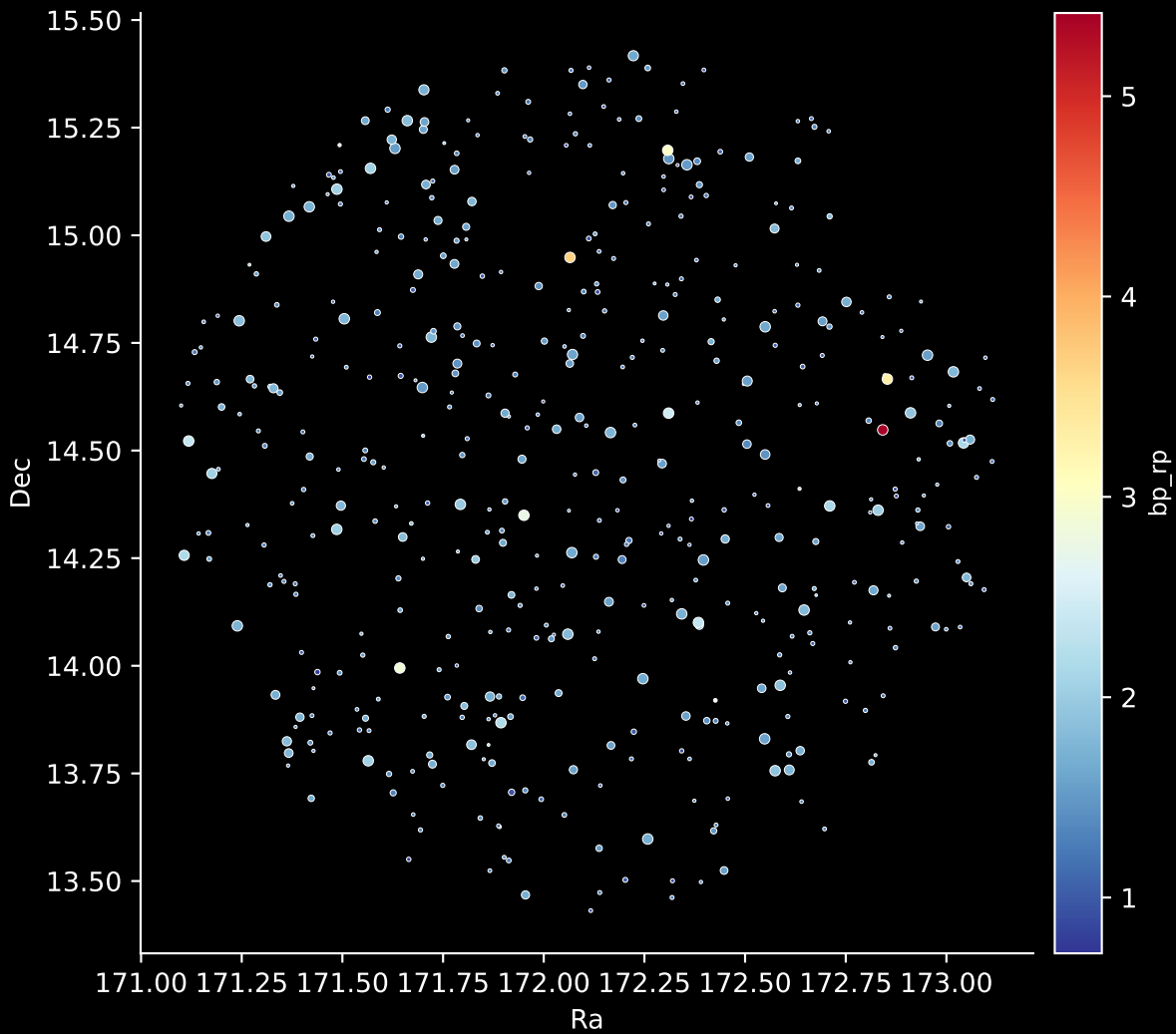
GALAH DR4 Field: [6785] Stars: 462
