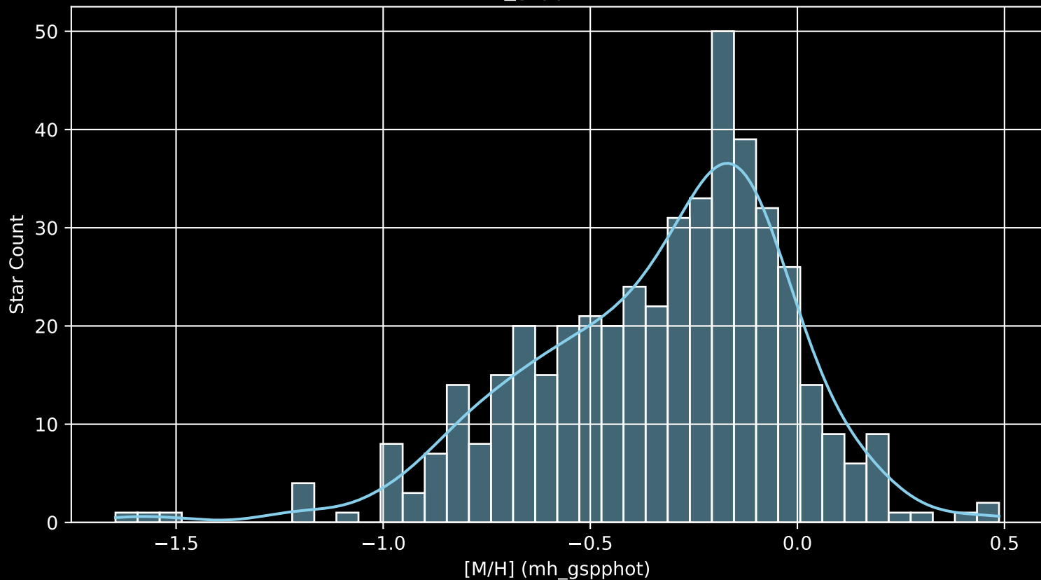
GALAH DR4 Field: [6785] [M/H] (mh_gspphot) (n= 459)
