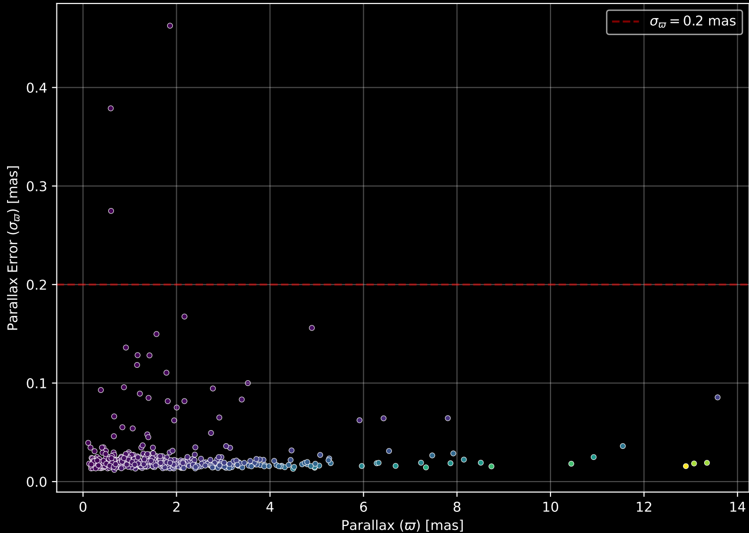
GALAH DR4 Field: [6785] Parallax Quality (n= 462)
